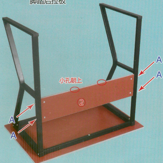
脚踏后拉板
